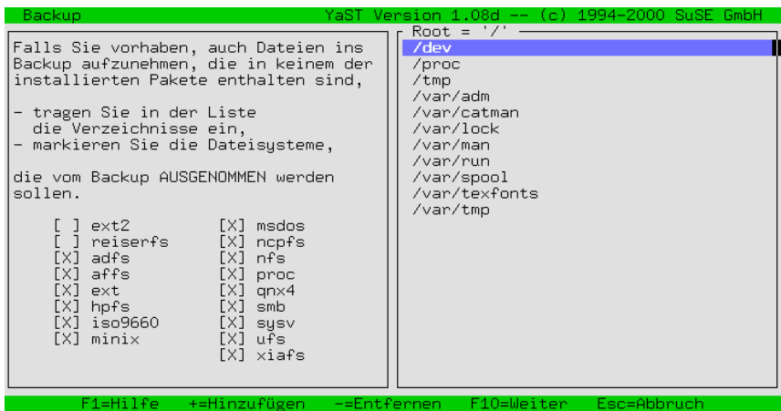
Abbildung 3.33: Datensicherung (Backup) mit YaST
