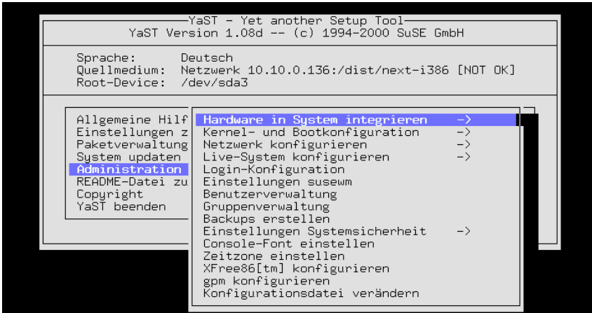
Abbildung 3.21: Administration des Systems
