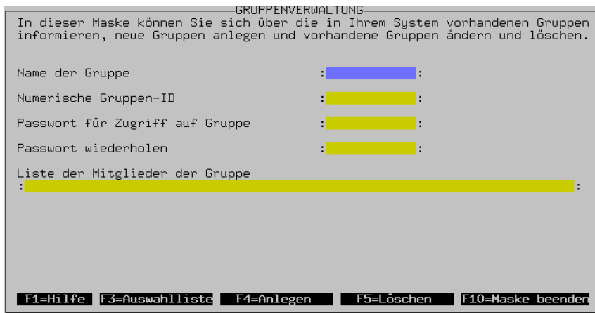
Abbildung 3.32: Gruppenverwaltung mit YaST
