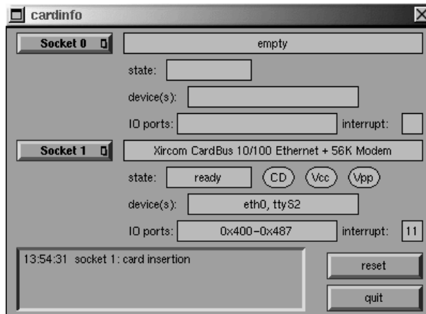
Abbildung 7.1: PCMCIA – Cardinfo
