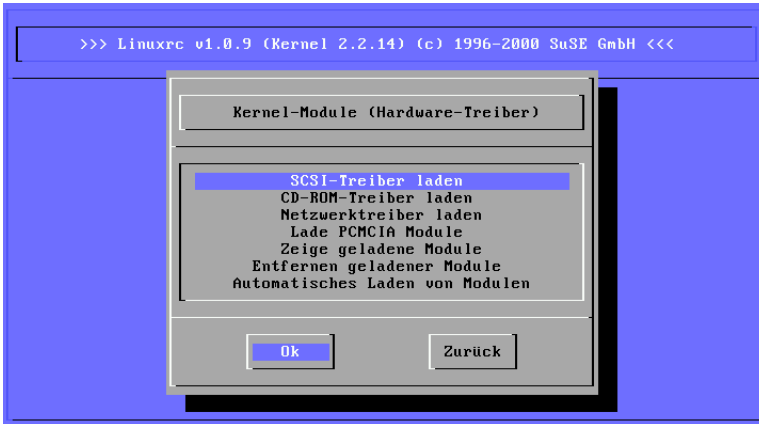
Abbildung 12.2: Module laden
