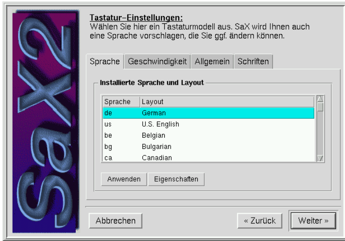
Abbildung 5.4: SaX2: Tastaturkonfiguration
