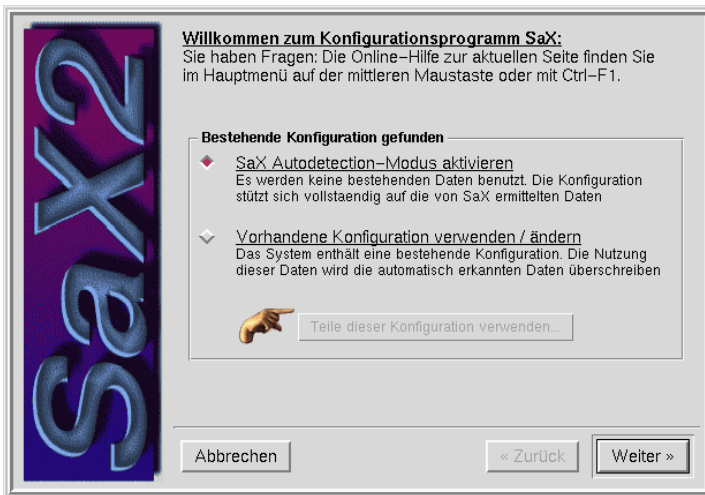
Abbildung 5.2: SaX2: Begrüßungsdialog
