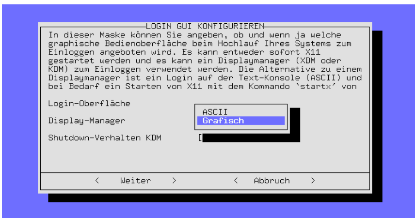
Abbildung 3.29: Login-Konfiguration
