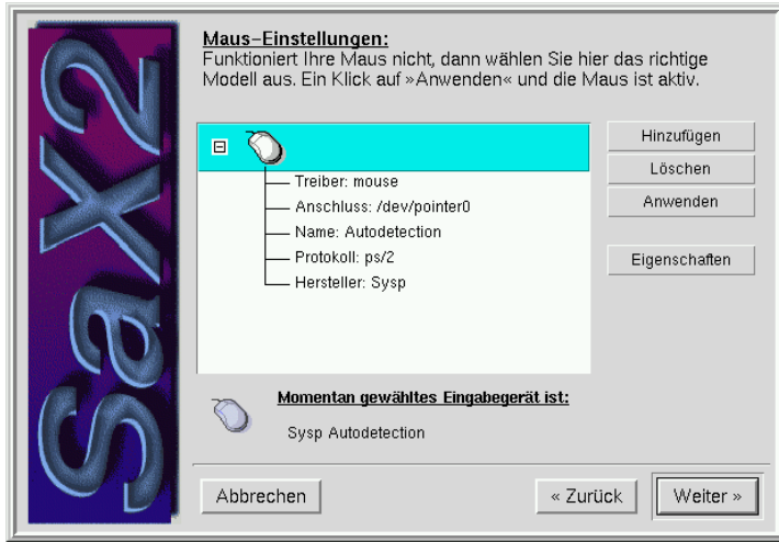
Abbildung 5.3: SaX2: Mauskonfiguration
