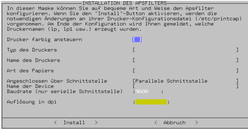
Abbildung 3.23: apsfilter mit YaST einrichten
