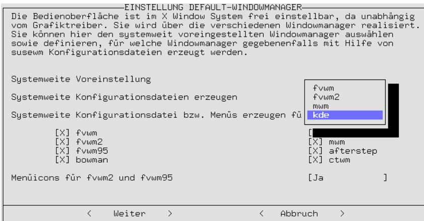
Abbildung 3.30: Einstellungen susewm
