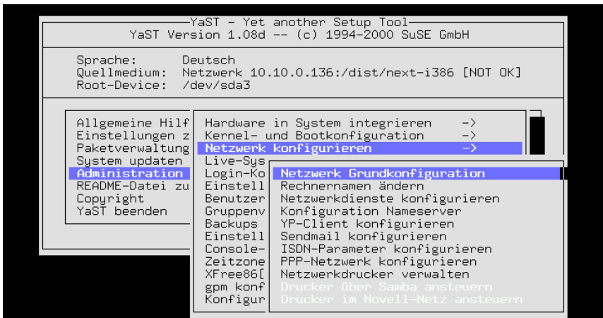
Abbildung 3.27: Netzwerk konfigurieren
