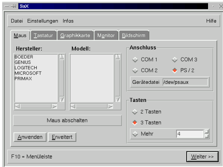
Abbildung 5.8: SaX: Mauseinstellungen
