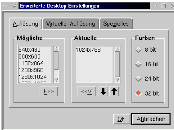
Abbildung 5.14: SaX: Bildschirm
