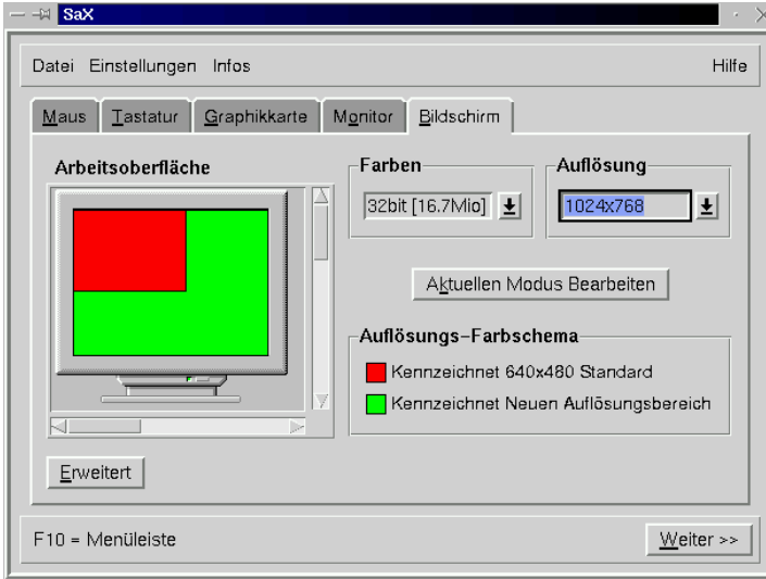
Abbildung 5.13: SaX: Bildschirm
