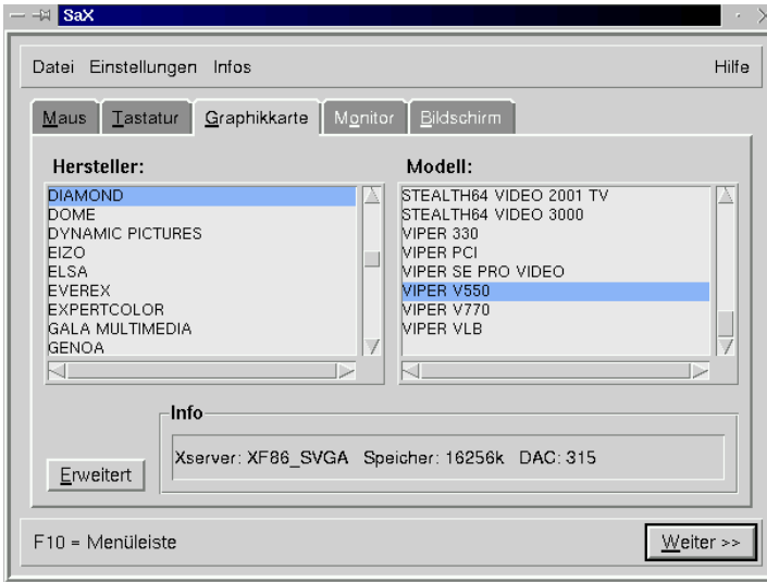
Abbildung 5.11: SaX: Grafikkarte
