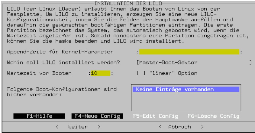
Abbildung 3.25: LILO: Installation
