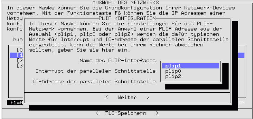
Abbildung 3.6: PLIP-Konfiguration
