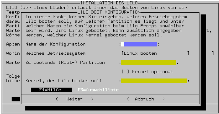
Abbildung 3.26: LILO: Bootkonfiguration
