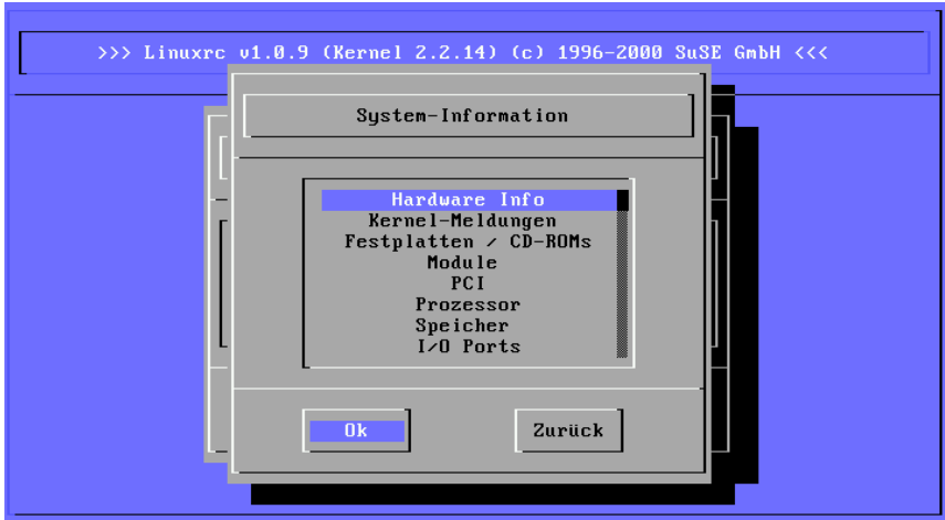
Abbildung 12.1: Systeminformationen
