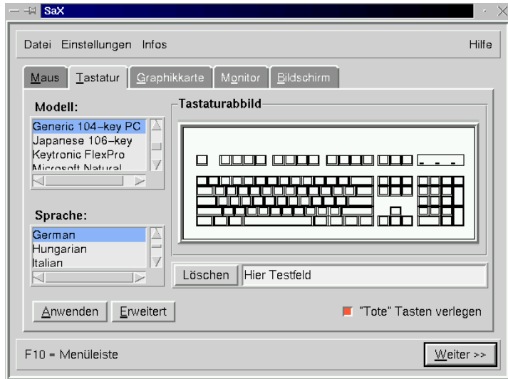
Abbildung 5.10: SaX: Tastatur
