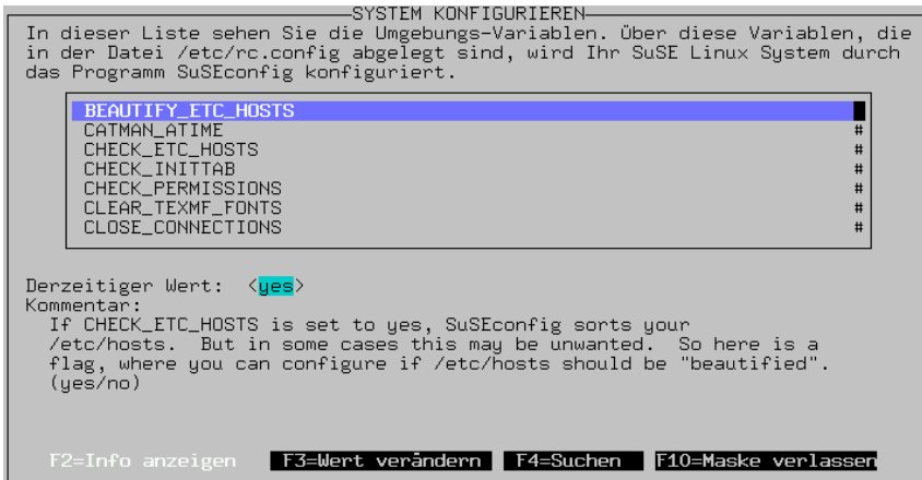
Abbildung 3.36: Verändern der Konfigurationsdatei mit YaST
