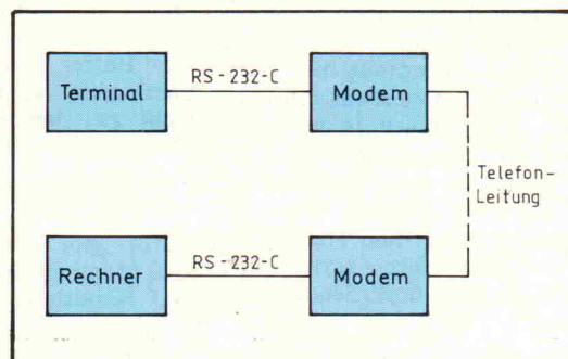
Bild 4. Terminalanschluß über RS-232-C und Modem
