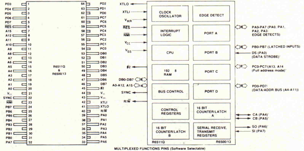
Pinbelegung
