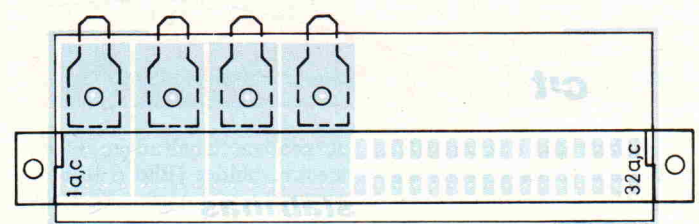
Bild 9. Bestückungsplan der Mikro-Busplatine
