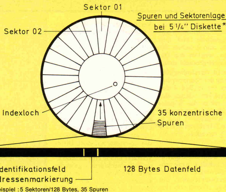
Bild 3. Das Soft-Sektor-Format bei 5 Sektoren pro Track
