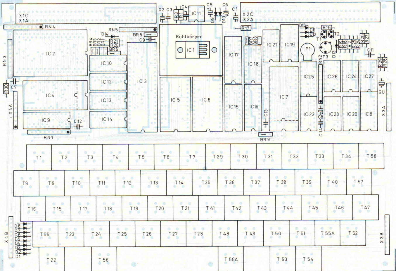
Bild 6. Bestückungsplan
