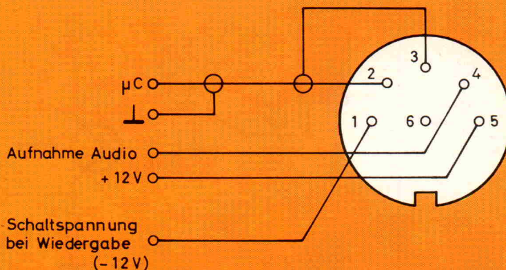
Bild 4. Belegung einer OIN-VCR- Buchse. Der von uns mit \mu\text{C} bezeichnete Pin wird mit dem Videoausgang des Rechners verbunden.
