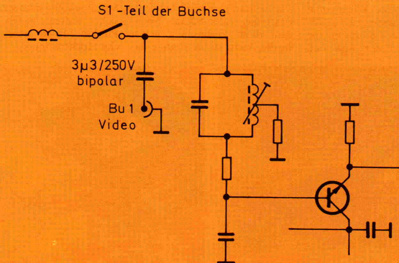
Bild 3. So muß die Schaltbuchse angeschlossen werden.
