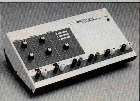
A-D-A-Konverter
